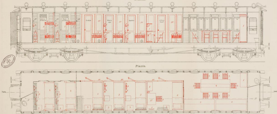
Carrozza di III cl. Ferrovie dello Stato - Serie CI, tipo 1907.
