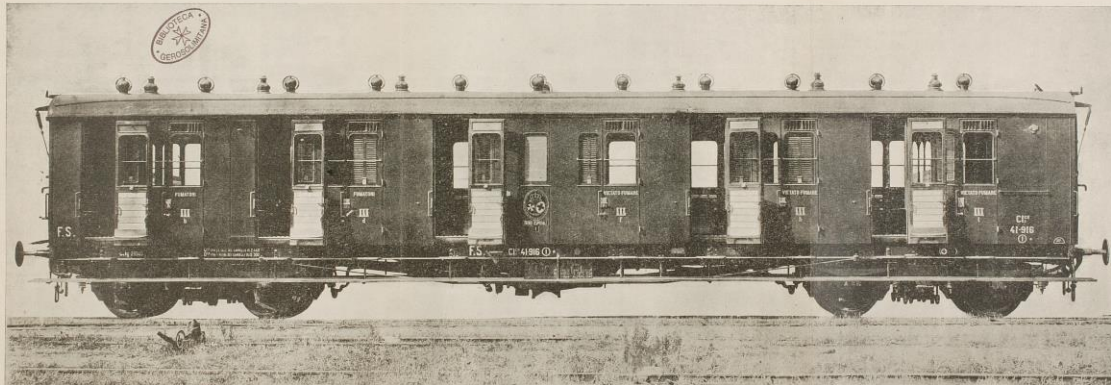
Carrozza Ferrovie Stato - Serie CI, 1910 ordinazione 1911.
