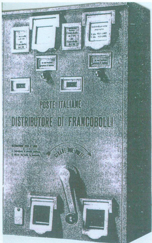
Riproduzione del distributore Autophon 283 a manovella adottato dalle Poste italiane nel 1975 ↓ francobolli distribuiti ↓
