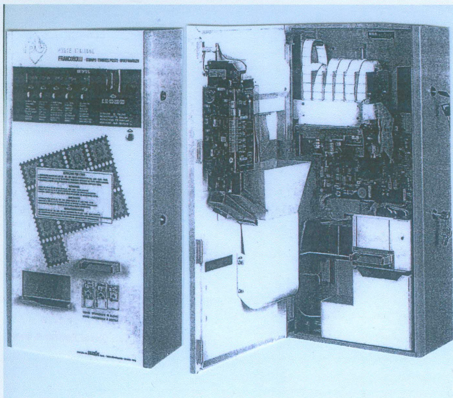
Esterno e interno del modello Afra/2 più pratico e " comunicativo " dei precedenti: le bobine in questa versione sono inserite nel corpo del distributore ↓ nuovi francobolli distribuiti oltre a quelli precedenti da Afra e Dafne ↓
