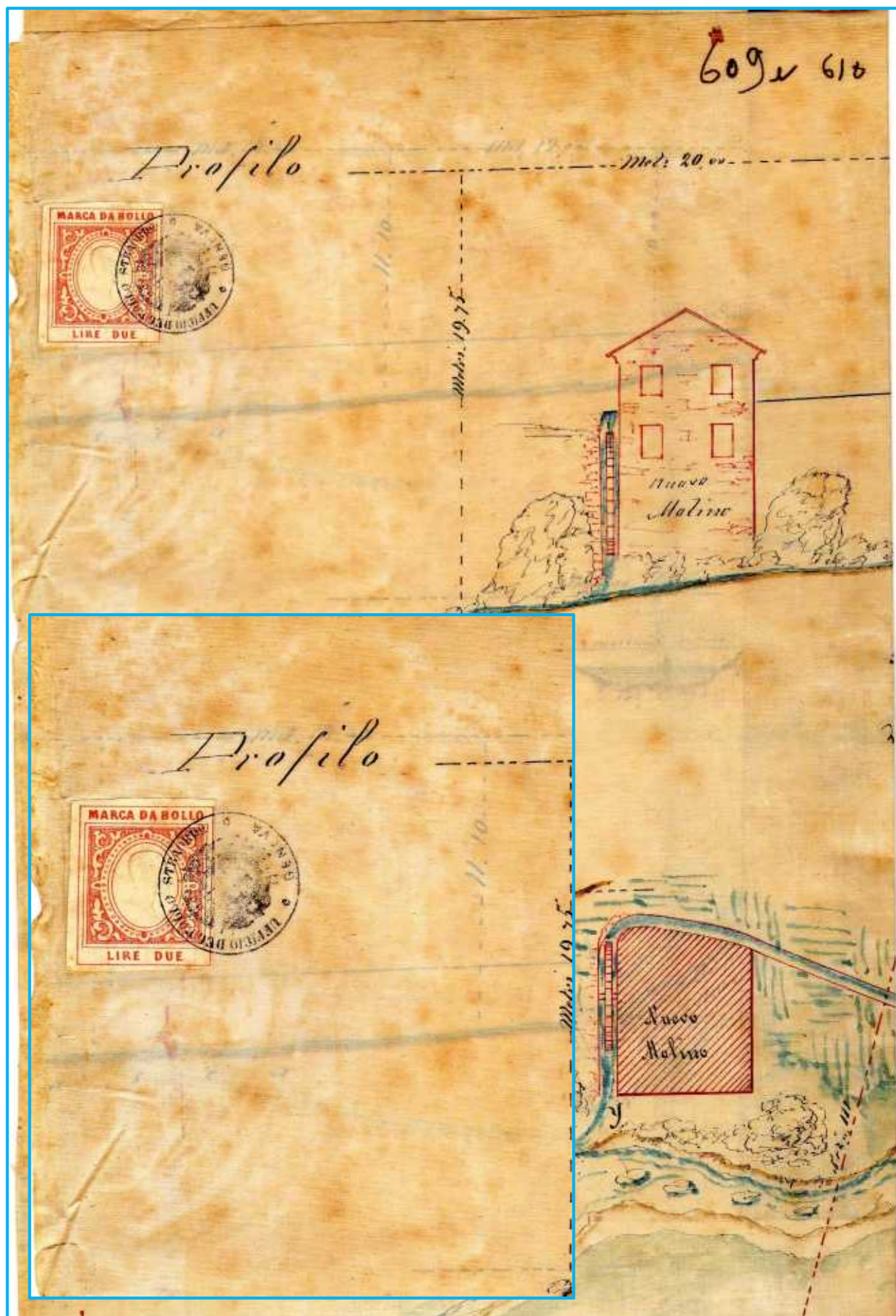
Progetto per mulino Genova 1 luglio 1863 – annullo dell'Ufficio del Bollo Straordinario – cm. 62x35,2
