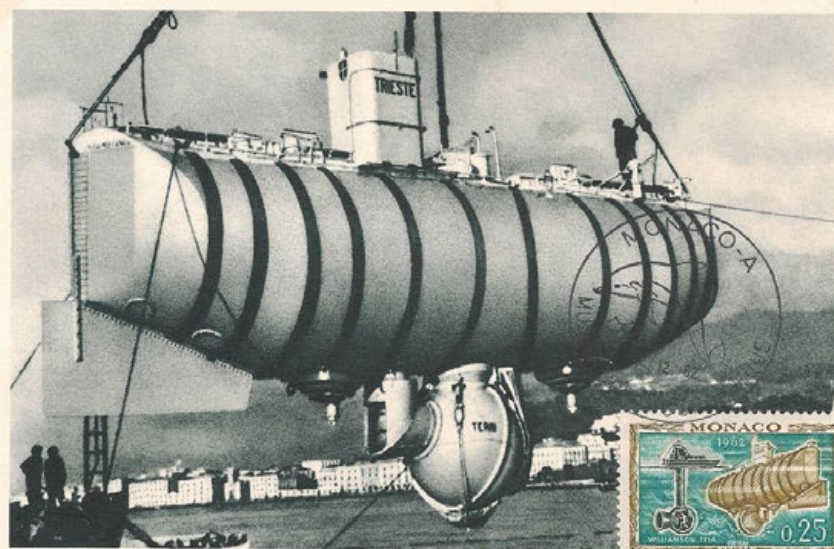
Bathyscaphe du Professeur Piccard : Le Trieste
