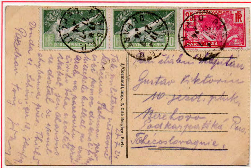
45 Cent - Auslandspostkarte
